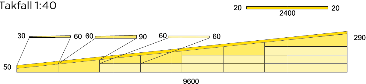
Takfall 1:40
